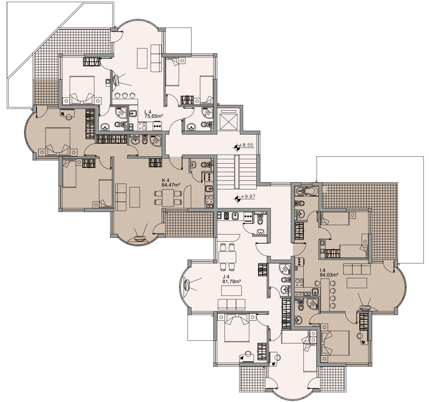
Съществуващо положение
