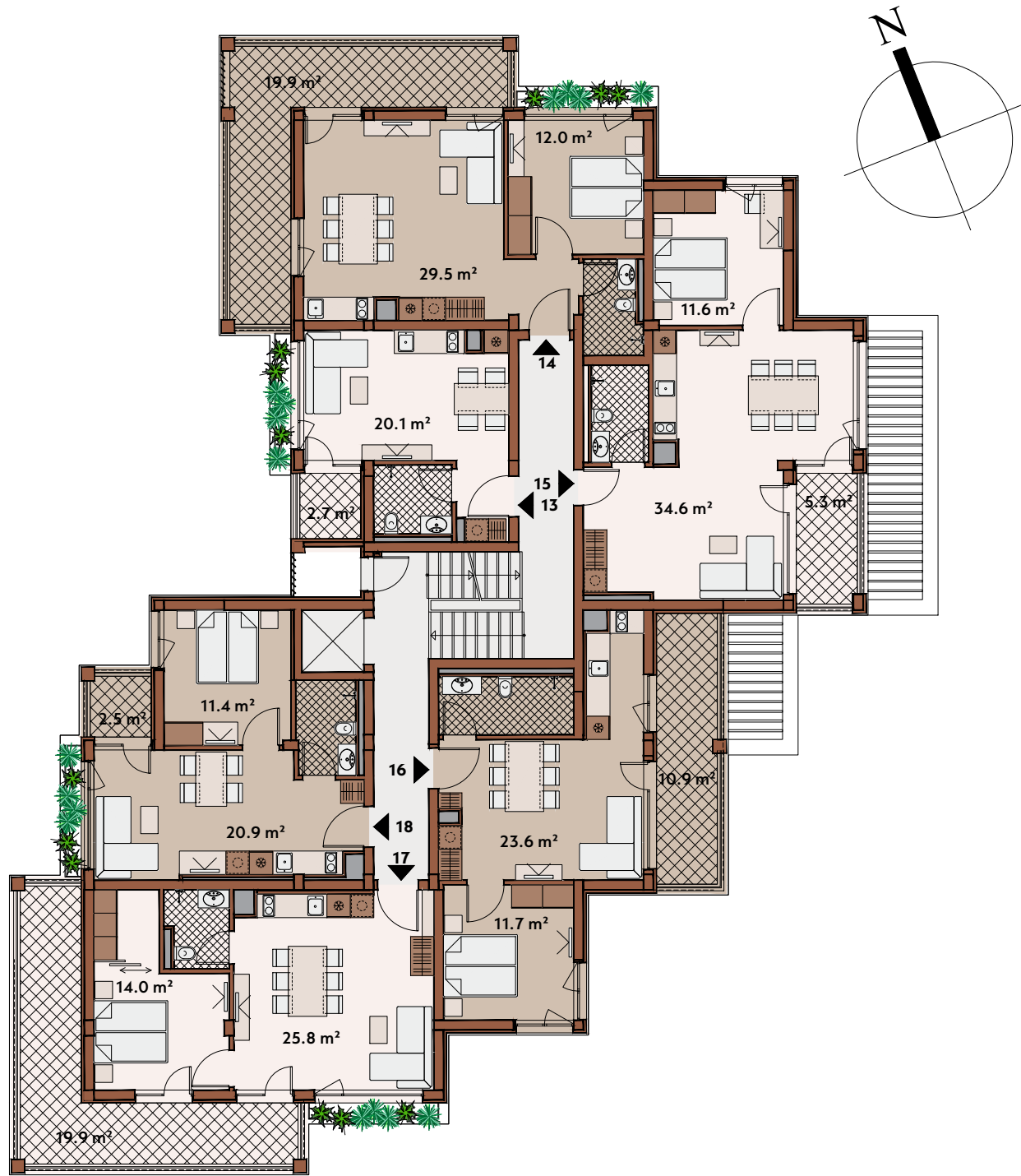
Проектно решение
