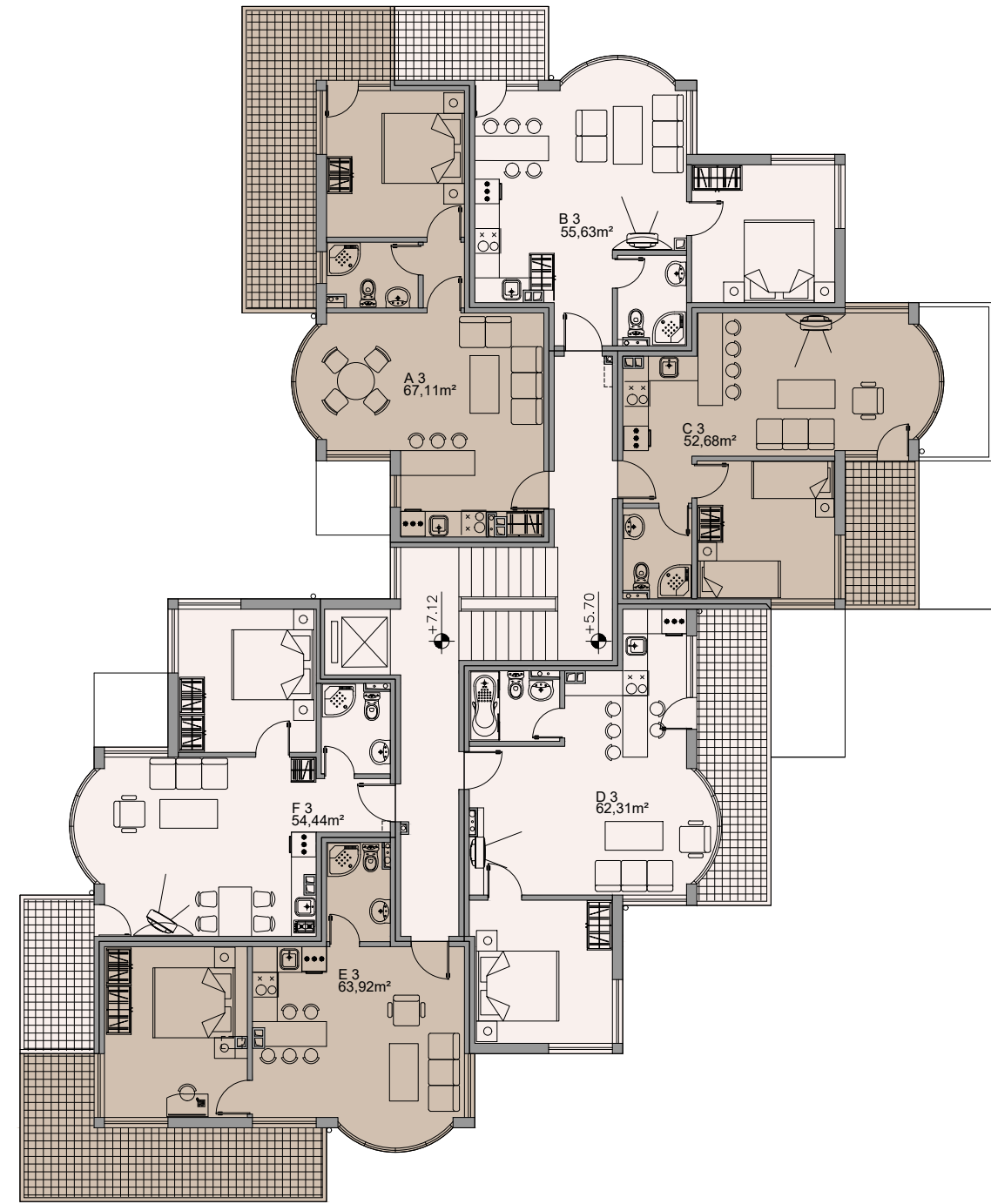
Съществуващо положение
