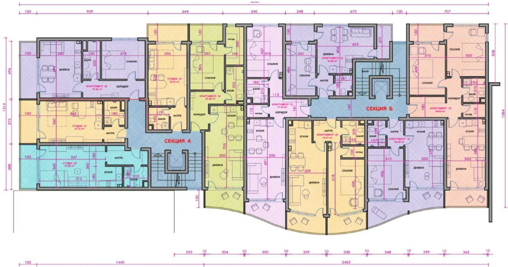
ПЕТИ ЕТАЖ (ЧЕТВЪРТИ ЖИЛИЩЕН) КОТА +11.80
