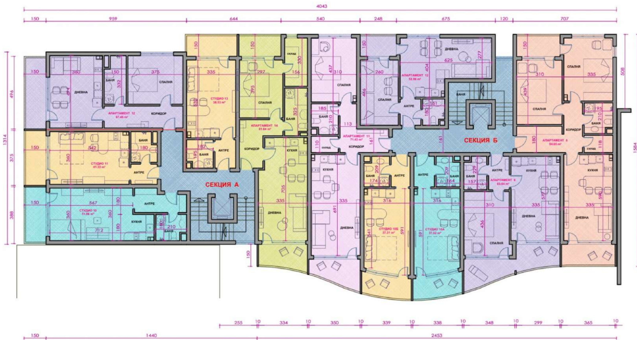
ТРЕТИ ЕТАЖ (ВТОРИ ЖИЛИЩЕН) КОТА +6.20
