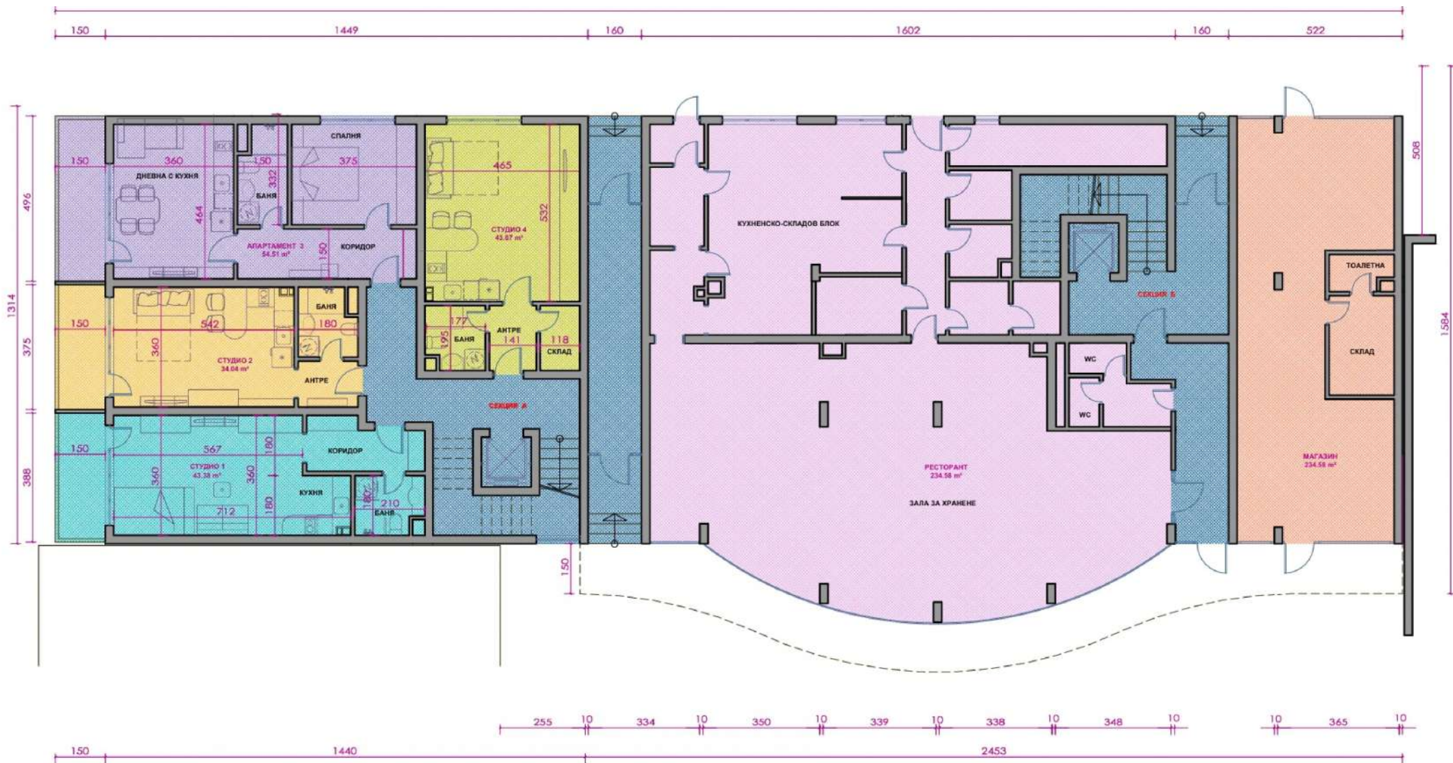
ПЪРВИ ЕТАЖ (ПАРТЕР) КОТА ±0.00
