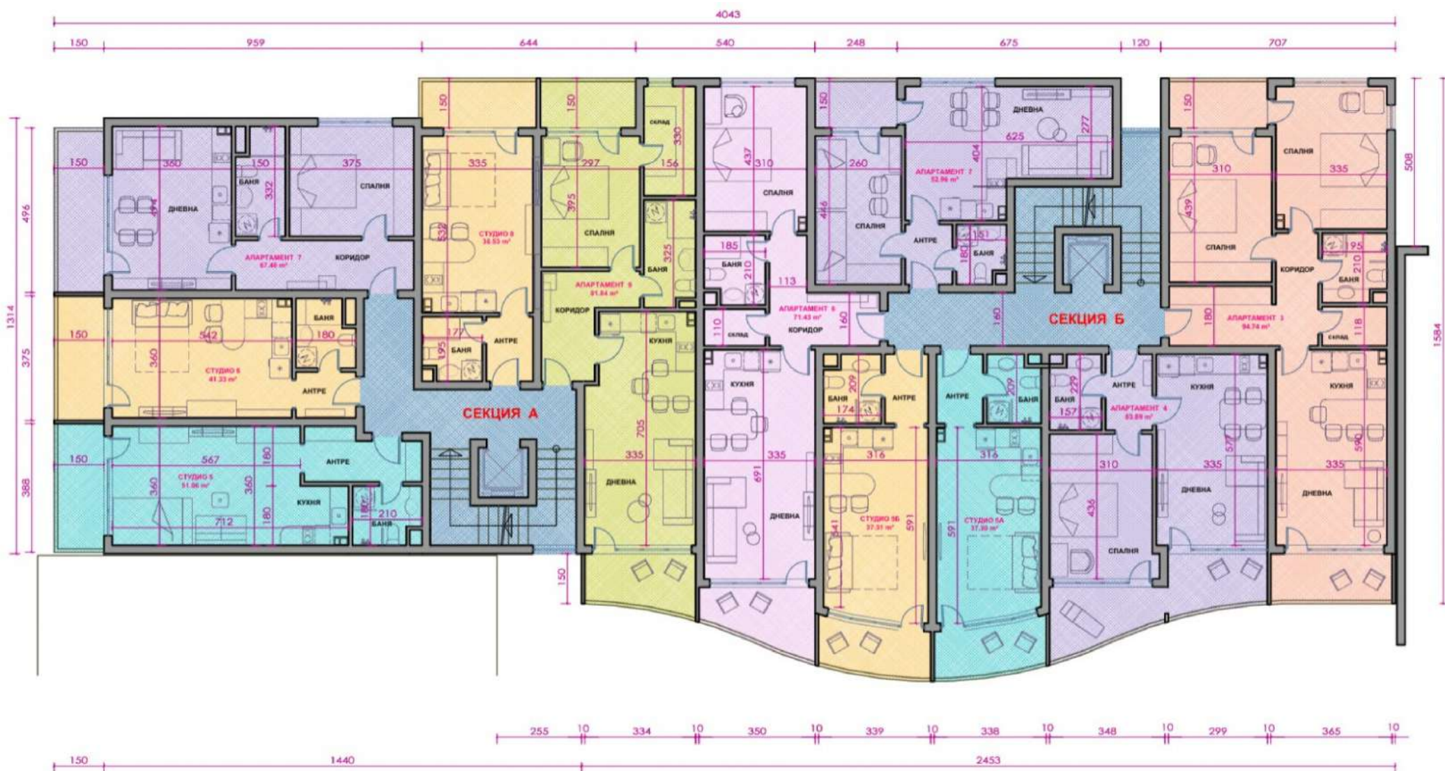
ВТОРИ ЕТАЖ (ПЪРВИ ЖИЛИЩЕН) КОТА +3.40
