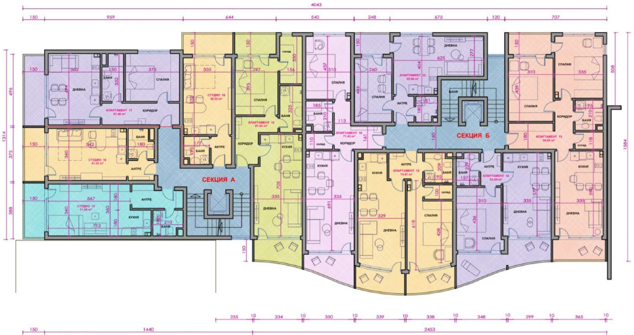
ЧЕТВЪРТИ ЕТАЖ (ТРЕТИ ЖИЛИЩЕН) КОТА +9.00
